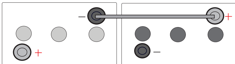
6 Volt 2 Pole Battery Blocks
